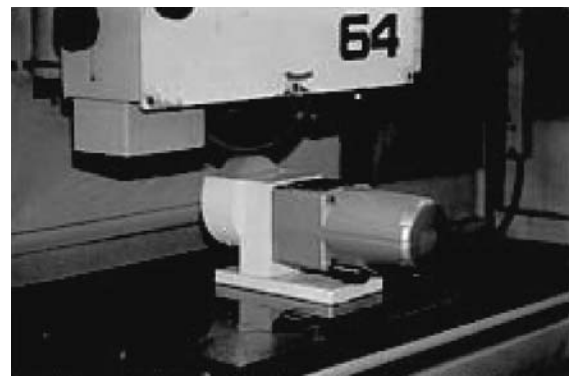
ダイヤモンド & CBN 平研用ツルーイング装置 TD-2
